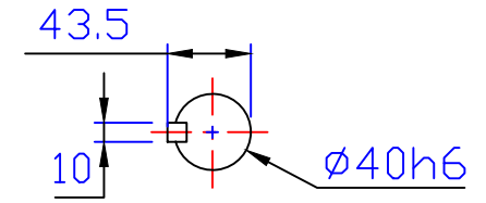
出力轴 Output Shaft
