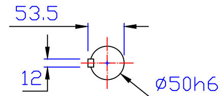
出力軸 Output Shaft
