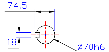
出力軸 Output Shaft
