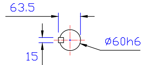
出力軸 Output Shaft
