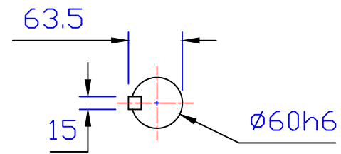
出力軸 Output Shaft
