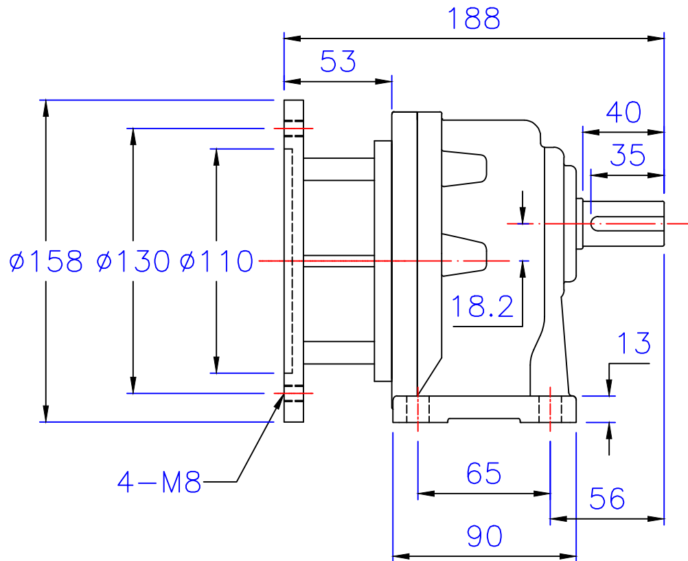
入力孔 Input hole
