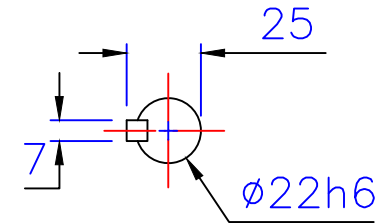
出力轴 Output shaft
