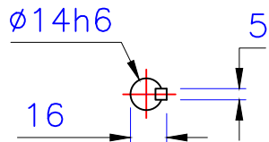
入力轴 Input shaft
