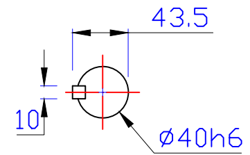
出力轴 Output Shaft
